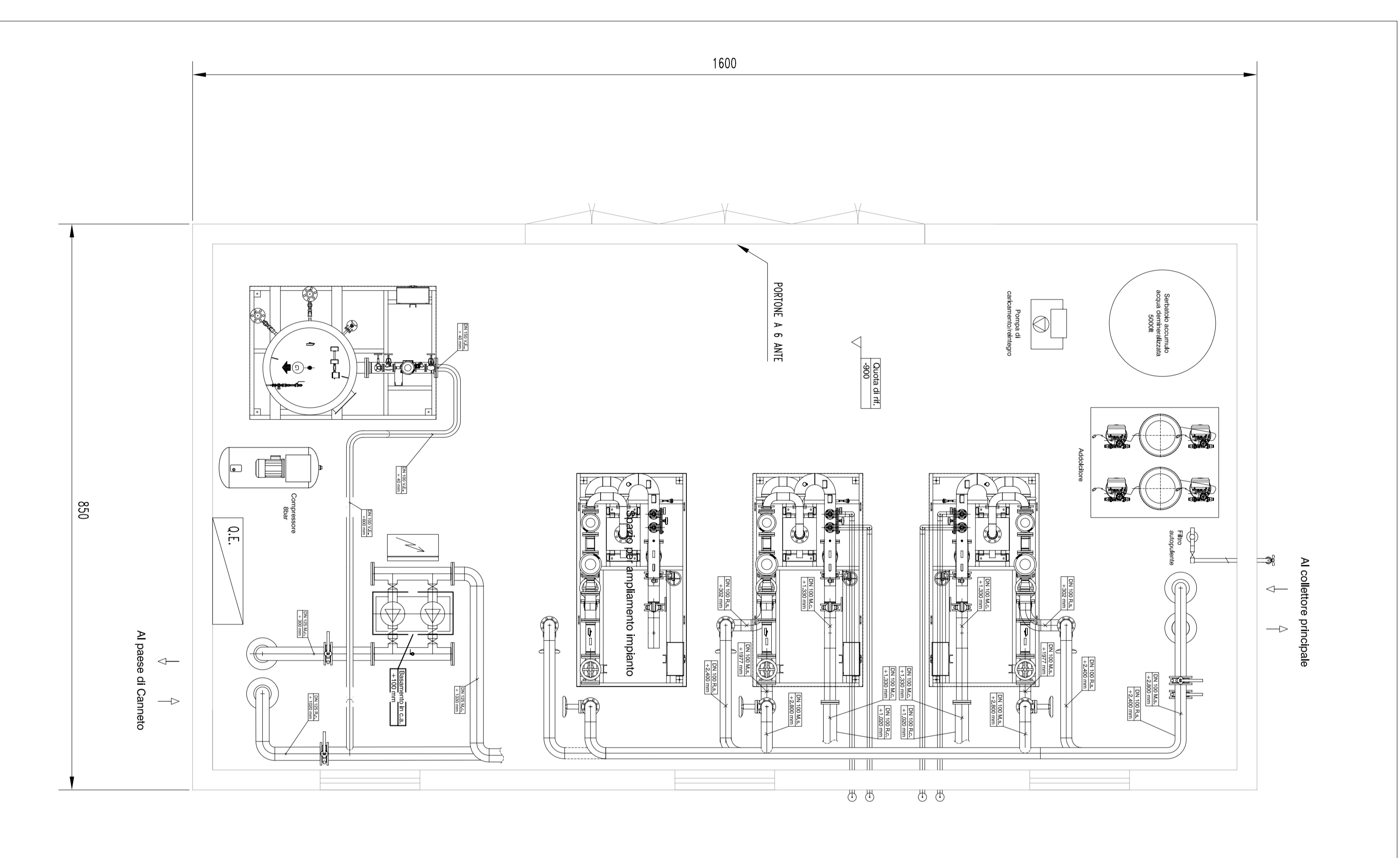
PLANIMETRIA GENERALE - CENTRALE "B"
