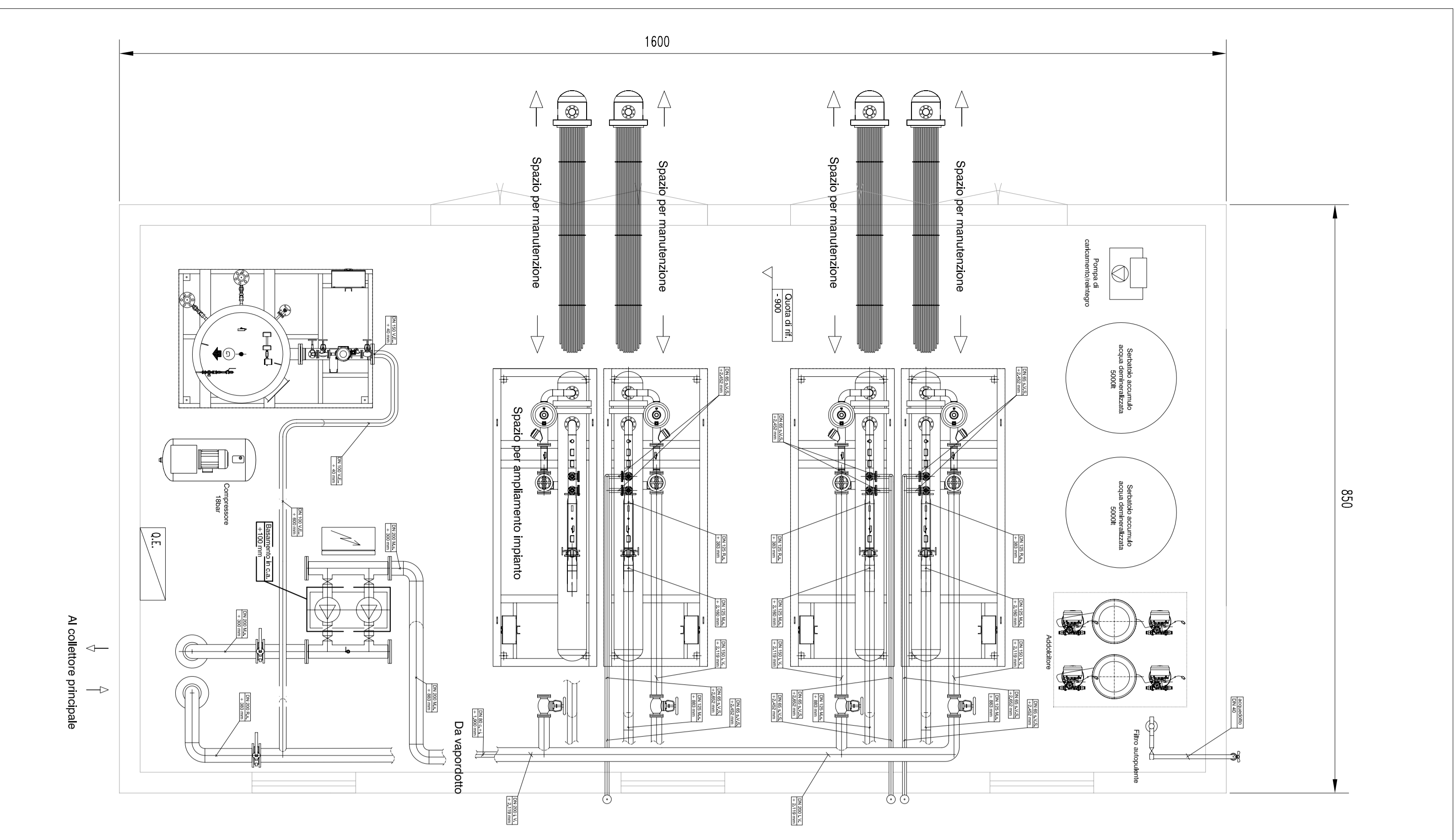
PLANIMETRIA GENERALE - CENTRALE "A"
