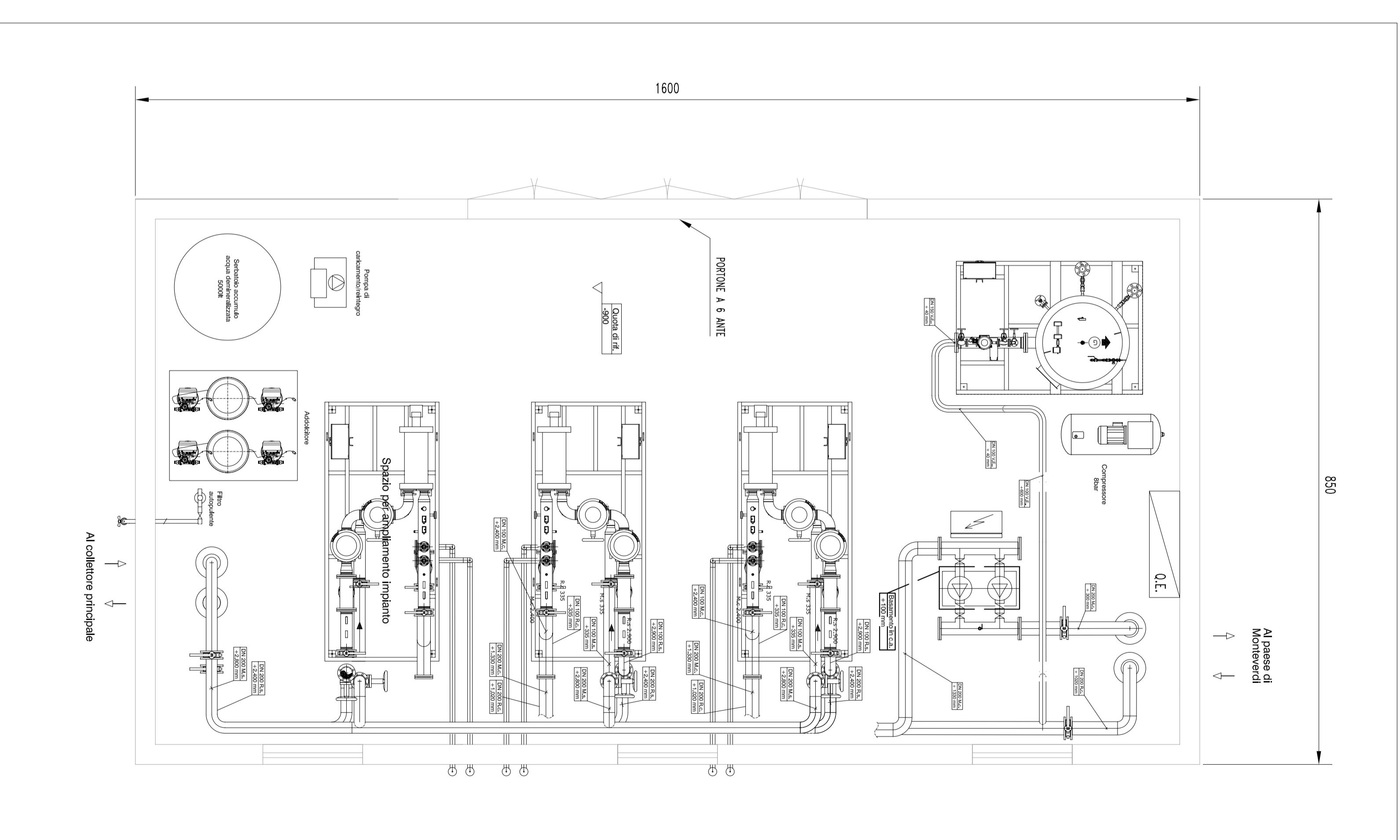
PLANIMETRIA GENERALE - CENTRALE "C"
